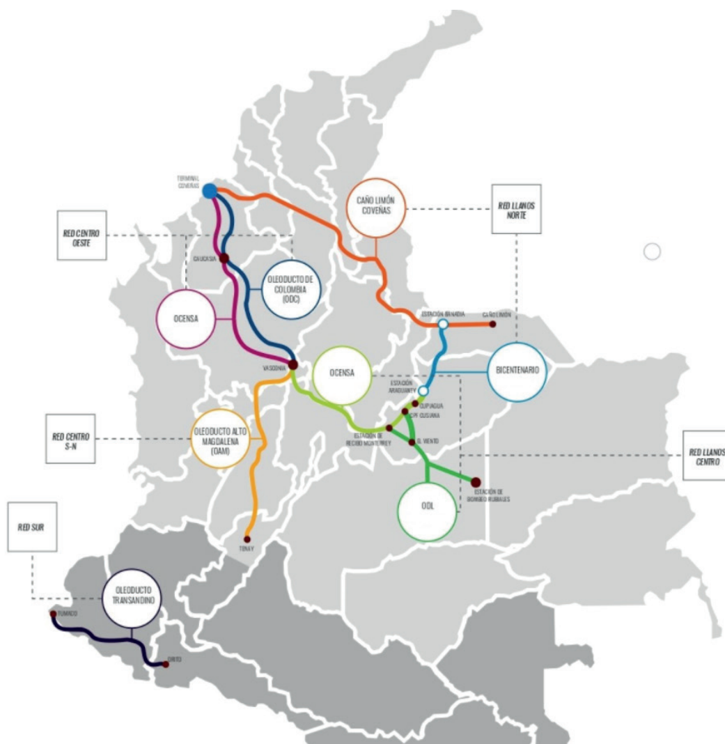
Ilustración 16. Red de Oleoductos Colombia
